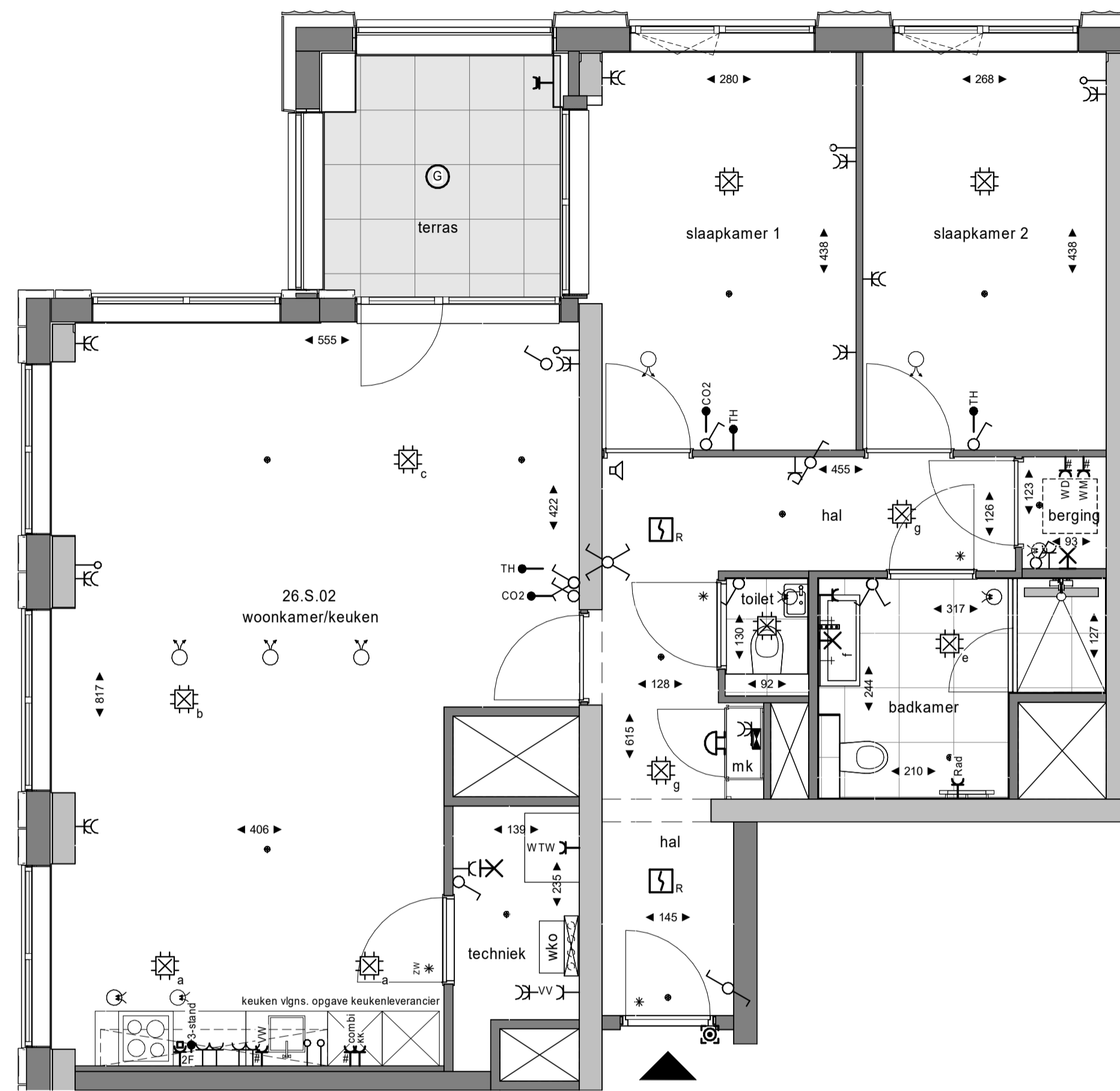
plattegrond 1 : 50 26e verdieping
